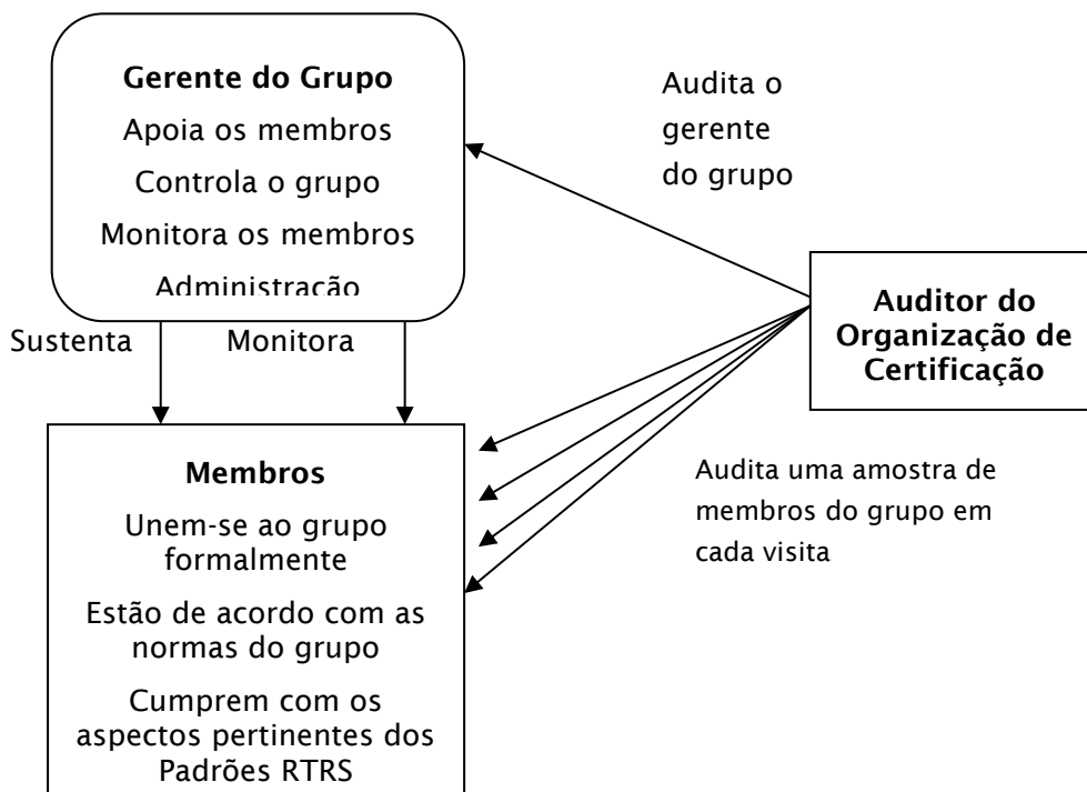
Figura 1. Certificação grupal
